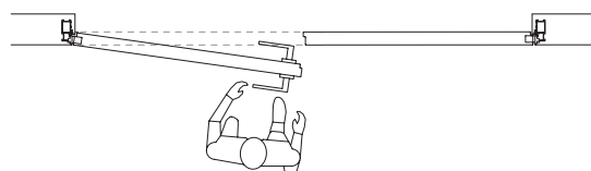
RIGHT PUSH DOOR - FIXED LEFT DOOR
